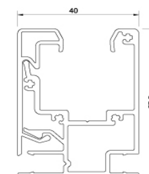
zusammenklappbare Führungsschiene
