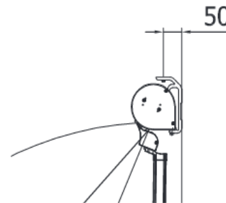
Deckenmontage
