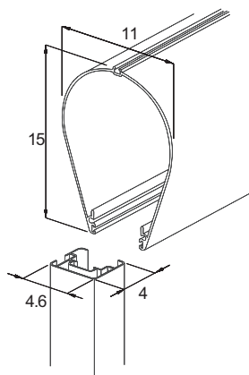
Abmessungen Schutzkasten und Führungsschiene
